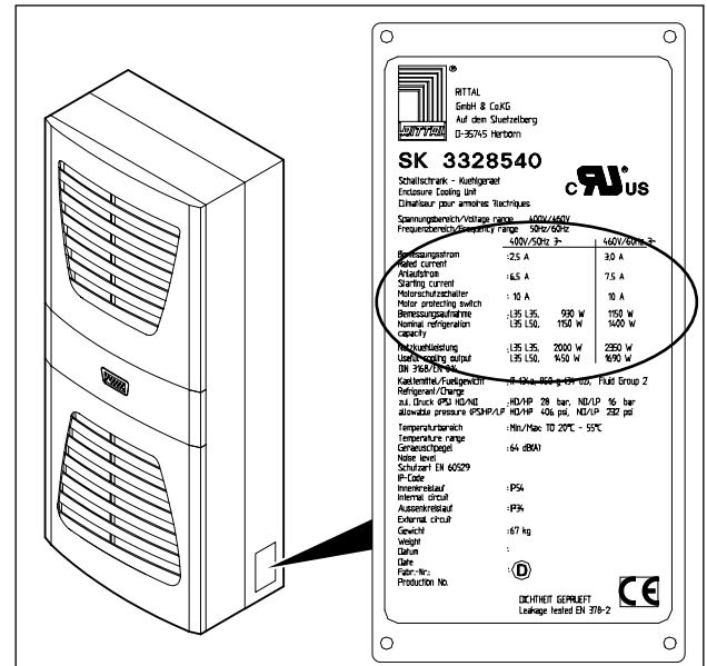
Imagen 84: Placa de características (Datos técnicos)
